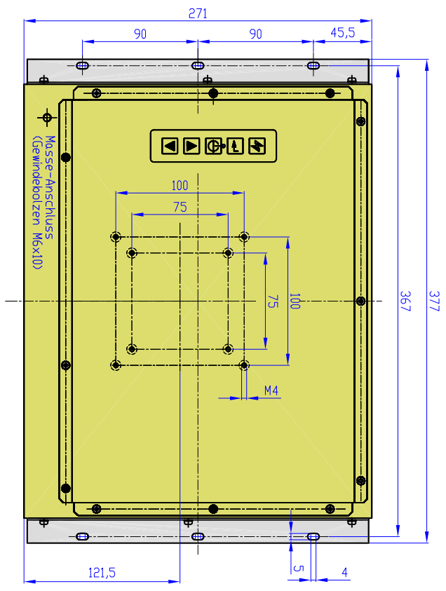
RÜCKANSICHT
